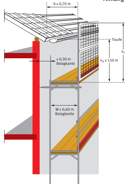
Bild 19: Abmessungen eines Dachfanggerüsts
